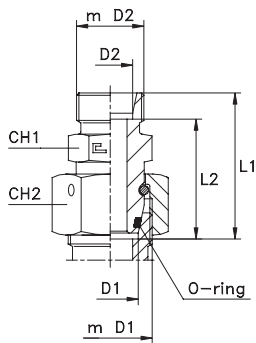
Typ: 6054...1 Körper
